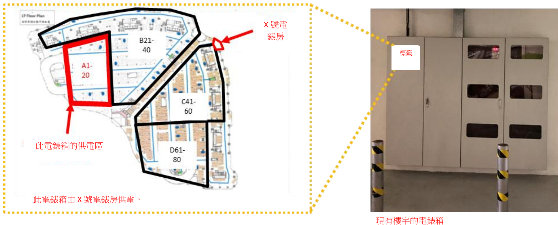
圖 4— 電動車充電設施供電區域平面圖示例
